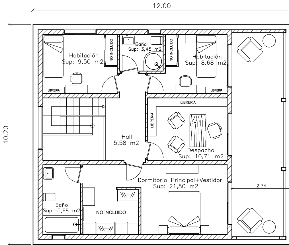
PLANTA ALTA
